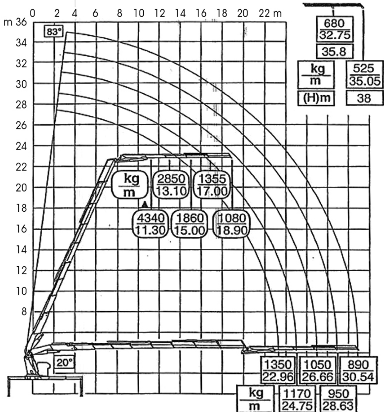
Diagramma di lavoro - con antenna
